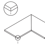
Cantos interiores Straight edge corners Angle intérieur Margelles bord intérieur arrondi Eckstufen Außenseite Внешний угол Angolo interno
