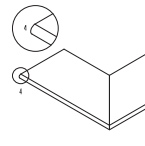
Cantos exteriores beilados Bullnose outer corners Margelles bord extérieur arrondi Abgerundete Außenseite (GRÜNG) Внешний угол с фаской Gradine con bordo esterno a toro
